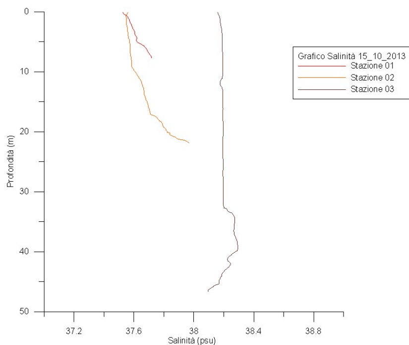
Fig. 6 Andamento della Salinità nelle Stazioni ST01PT, ST02PT, ST03PT durante le campagne FPOA_1
