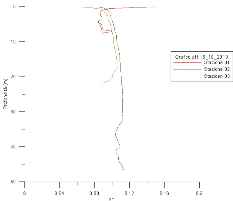
Fig. 7 Andamento della pH nelle Stazioni ST01PT, ST02PT, ST03PT durante le campagne FPOA_1
