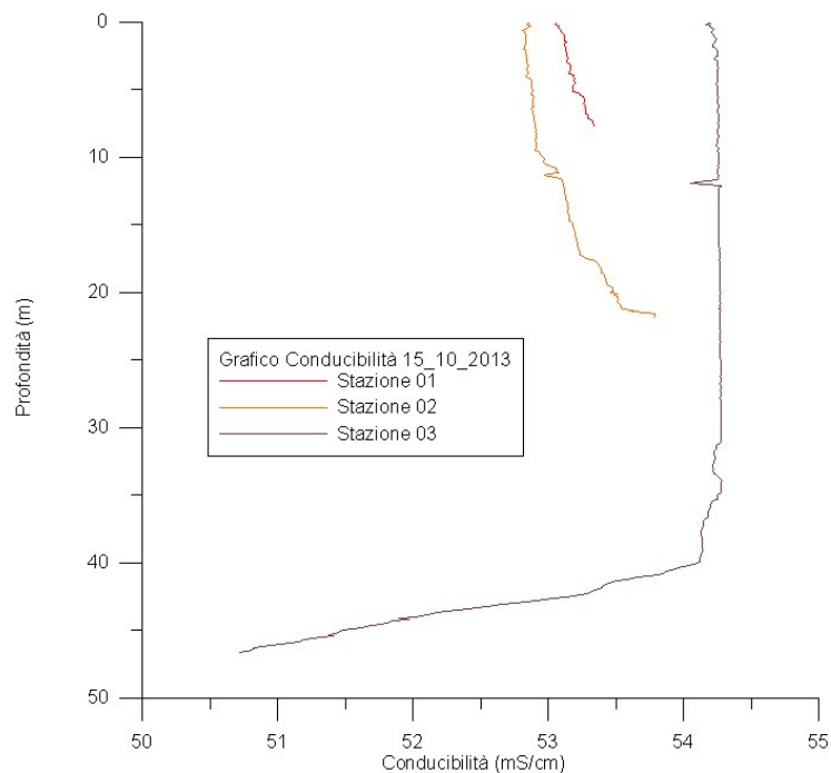
Fig. 5 Andamento della Conducibilità nelle Stazioni ST01PT, ST02PT, ST03PT durante le campagne FPOA_1
