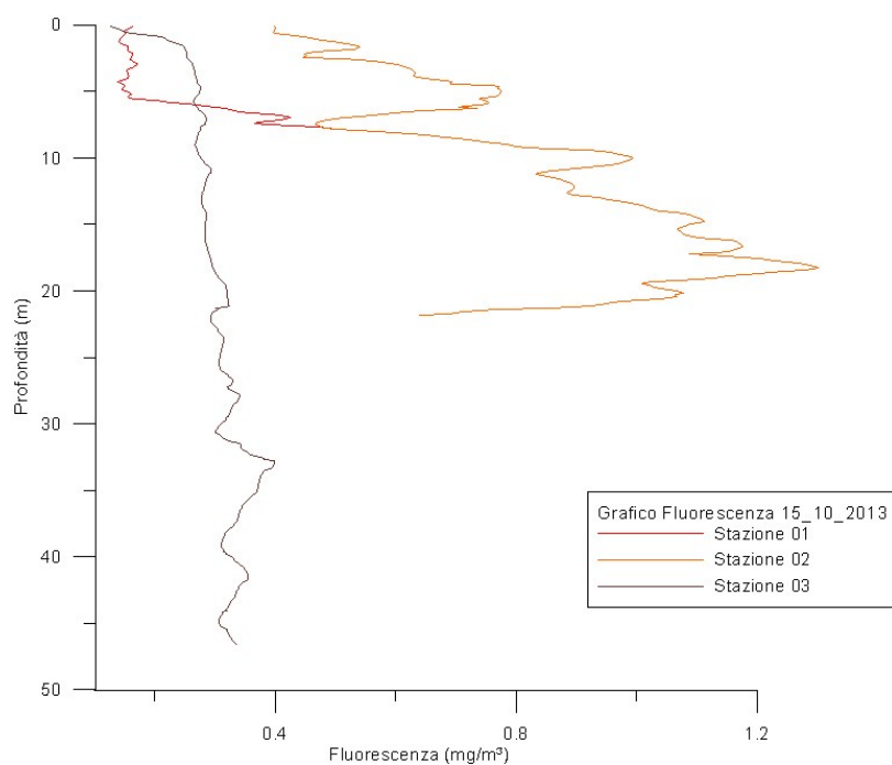
Fig. 9 Andamento della Clorofilla a nelle Stazioni ST01PT, ST02PT, ST03PT durante le campagne FPOA_1
