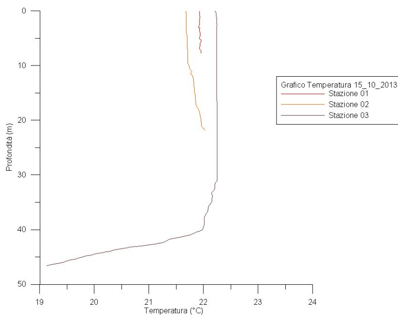
Fig. 4 Andamento della Temperatura nelle Stazioni ST01PT, ST02PT, ST03P durante le campagne FPOA_1
